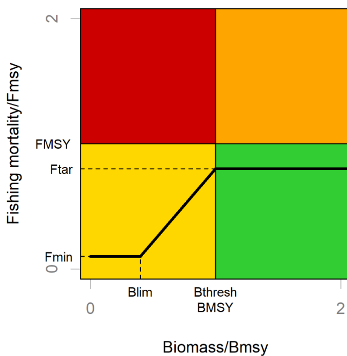
ALB-Figura 9. Forma gráfica de la HCR adoptada en la Rec. 17-04. B_{lim} (establecido en 0,4 B_{RMS} ) es el punto de referencia límite de la biomasa, B_{thresh} (establecido en B_{RMS} ) es el punto por debajo del cual la mortalidad por pesca desciende linealmente, F_{tar} (establecido en 0,8 F_{RMS} ) es la tasa de mortalidad por pesca objetivo que se tiene que aplicar para lograr los objetivos de ordenación, y F_{min} (establecido en 0,1 F_{RMS} ) es la mortalidad por pesca que se tiene que aplicar cuando B < B_{lim} .
