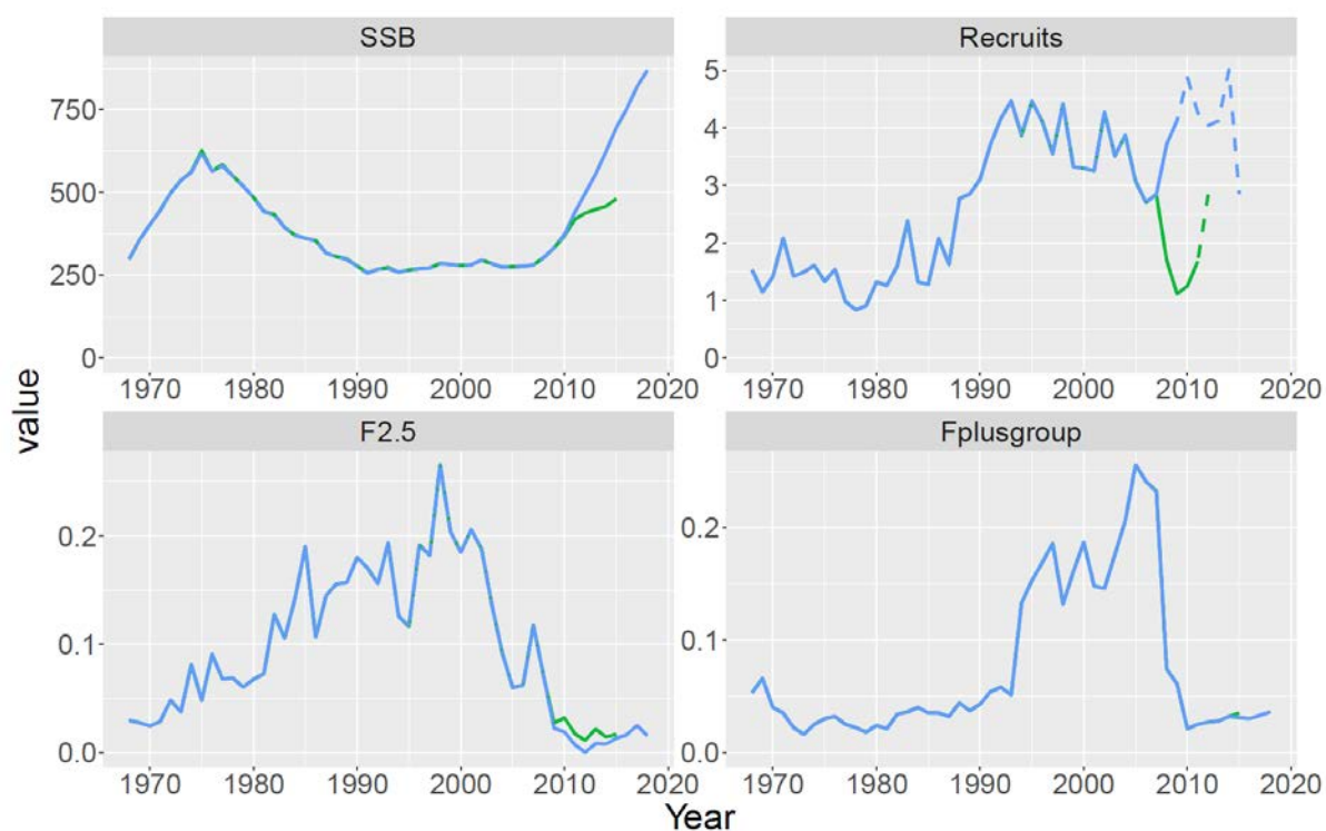
BFTE-Figura 3. Estimaciones de biomasa del stock reproductor (en miles de toneladas), reclutamiento (en millones) y mortalidad por pesca (media de las edades 2 a 5 y 10+) a partir del caso base del VPA en la evaluación de stock de 2020 (azul) en comparación con la evaluación del stock de 2017 (verde) para el periodo entre 1968 y 2015. Los reclutamientos de los últimos años (línea discontinua: 2012-2013 para la evaluación del stock de 2017 y 2010-2015 para la evaluación del stock de 2020) fueron pobremente estimados.
