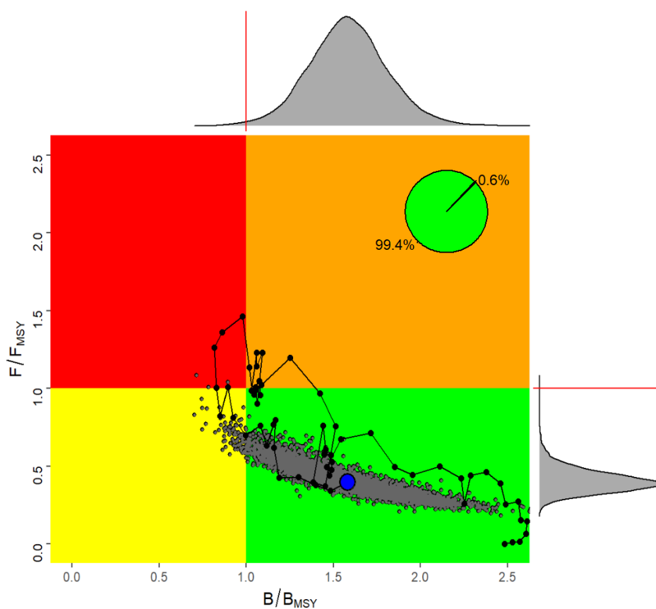
ALB-Figura 6. Atún blanco del Atlántico sur (diagrama de Kobe). Trayectorias del estado del stock de B/B_{MSY} y F/F_{MSY} a lo largo del tiempo (1956-2018), así como la incertidumbre (puntos grises) en torno a la estimación actual (2018) (punto azul) basadas en el modelo de producción excedente bayesiano con la probabilidad de estar sobrepescado y sufriendo sobrepesca (rojo, 0 %), de no estar ni sobrepescado ni sufriendo sobrepesca (verde, 99,4 %) y de estar sobrepescado (amarillo, 0,6 %).
