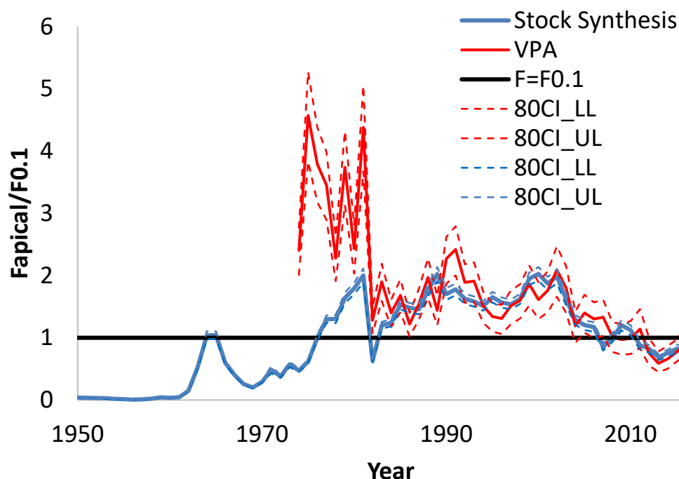
BFTW-Figura 3. Mortalidad por pesca en relación con el punto de referencia F_{0.1} estimada por el VPA (rojo) y el Stock Synthesis (azul) para la evaluación de 2020. Los intervalos de confianza del 80 % se indican con líneas discontinuas.
