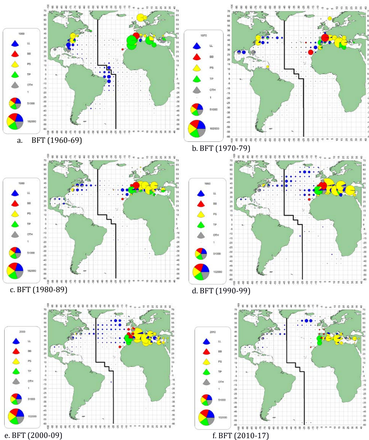
BFT-Figura 1. Distribución geográfica de las capturas de atún rojo por cuadrículas de 5x5 y por artes principales desde 1960 a 2017 (la última década solo cubre 8 años).
