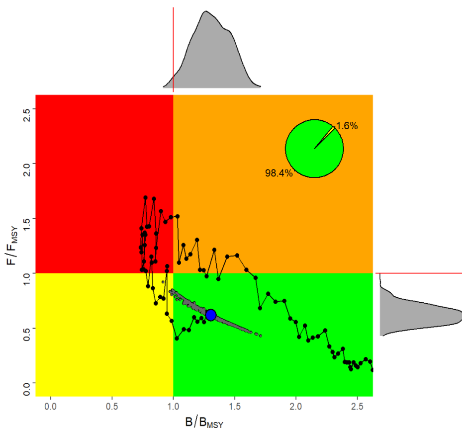
ALB-Figura 4. Atún blanco del Atlántico norte (diagrama de Kobe). Trayectorias del estado del stock de B/B_{MSY} y F/F_{MSY} a lo largo del tiempo (1930-2018), así como incertidumbre (puntos grises) en torno a la estimación actual ( F_{2018}/F_{MSY} , B_{2018}/B_{MSY} ) (punto azul) basadas en el modelo de producción excedente con la probabilidad de estar sobrepescado y sufriendo sobrepesca (rojo, 0 %), de no estar ni sobrepescado ni sufriendo sobrepesca (verde, 98,4 %) y de estar sobrepescado (amarillo, 1,6 %).
