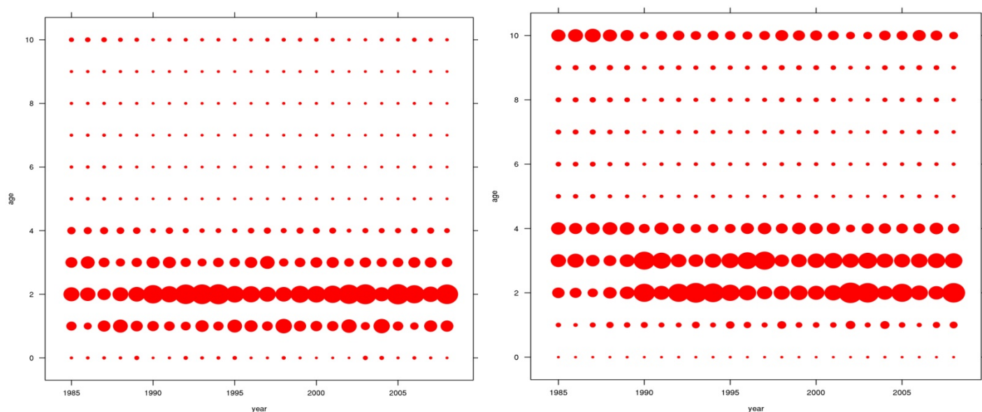
SWO-MED-Figura 6. Proporción de números de la captura (izquierda) y peso de la captura (derecha) por edad por año.
