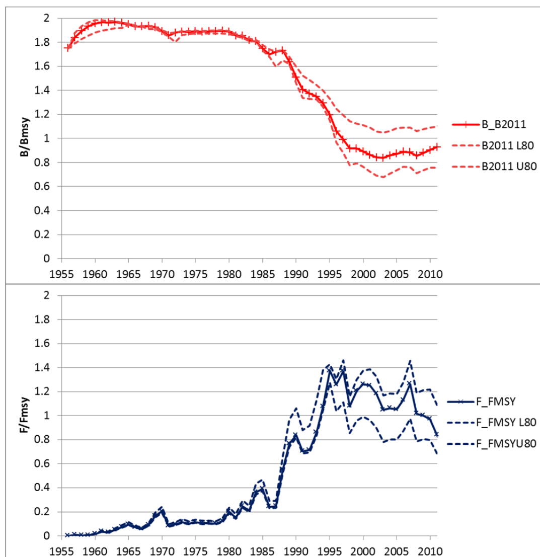
SWO-ATL-Figura 13. B/B_{MSY} y F/F_{MSY} estimadas para el pez espada del Atlántico sur a partir de ASPIC, la línea discontinua indica los límites del 80% inferiores y superiores de los ensayos de bootstrap.
