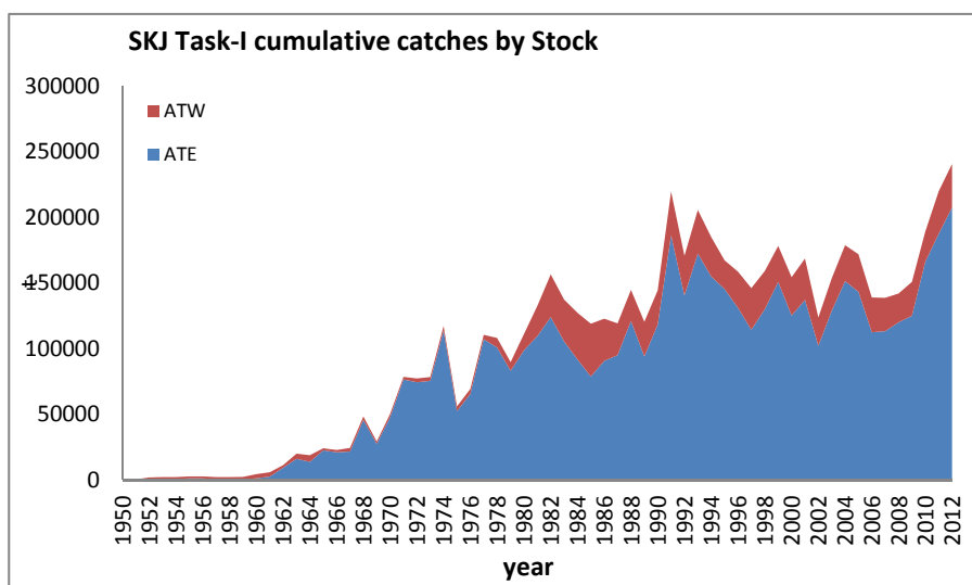
SKJ-Figura 2. Captura total (t) de listado en el Atlántico total y por stocks (Este y Oeste) entre 1950 y 2012. Las estimaciones de listado en el “ faux poisson ” desembarcado en Côte d’Ivoire fueron incluidas en las capturas comerciales de listado en el Atlántico este (para la evaluación sólo se ha considerado la captura hasta 2006). Es posible que las capturas de listado realizadas en el Atlántico este durante estos últimos años no hayan sido declaradas o que hayan sido subestimadas durante los procedimientos de corrección de la composición específica de los cuadernos de pesca basada en los muestreos multiespecíficos realizados en los puertos.
