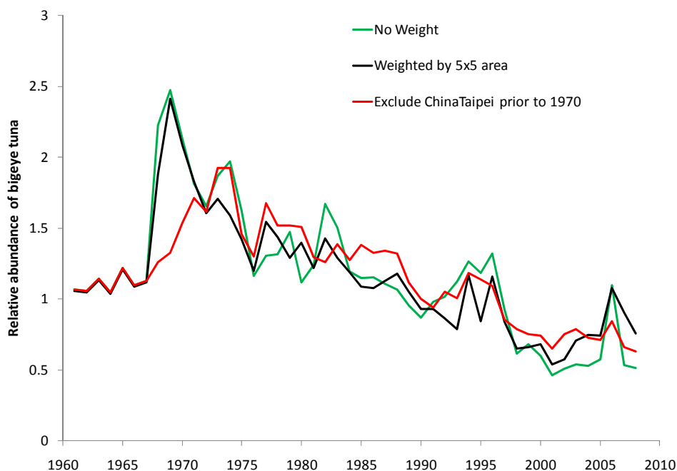
BET-Figura 5. Tres índices alternativos combinados seleccionados para la evaluación con modelos de producción logísticos en no equilibrio.
