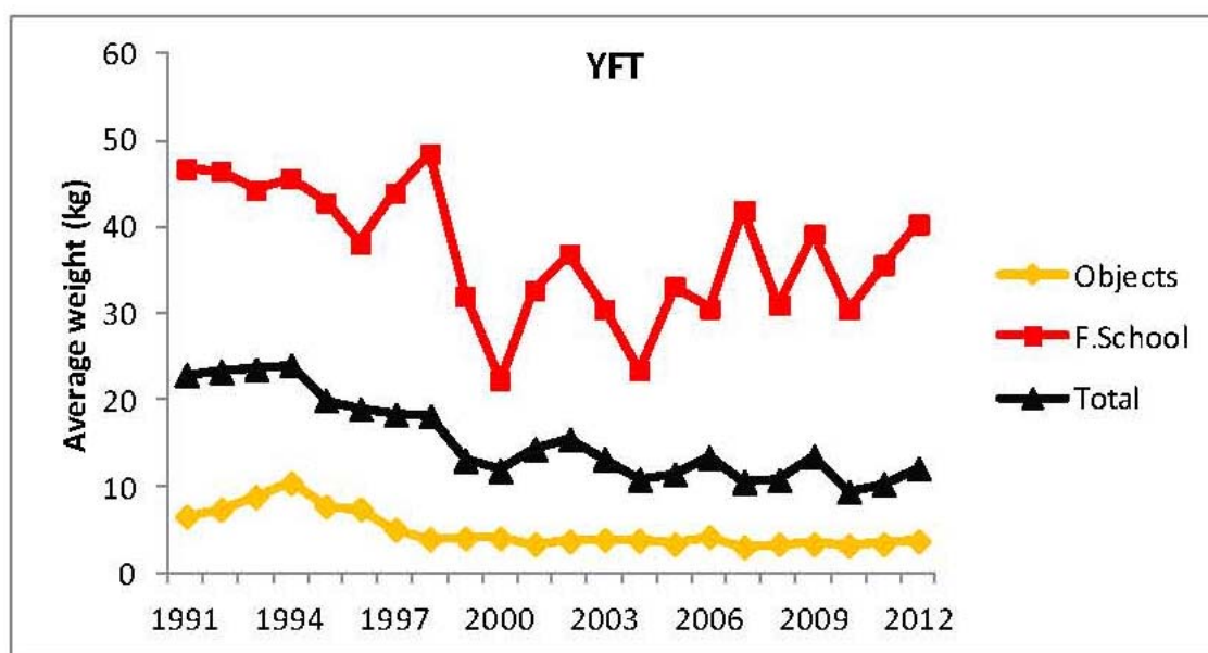
YFT-Figura 7. Tendencia del peso medio para el rabil basada en los datos de captura por talla a) por pesquerías principales (1970-2012) (Nota: los valores de 2011 y 2012 son preliminares basados en algunas series de CAS declaradas) y b) para los cerqueros europeos (total) y separada entre bancos libres y bancos asociados a DCP (1991-2012).
