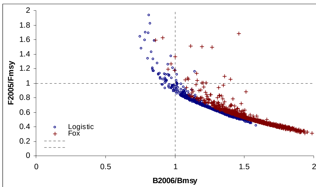
SWO-ATL Figura 6. Gráfico de dispersión de los pares estimados de ratios actuales de biomasa y mortalidad por pesca para el pez espada del Atlántico sur. Los resultados se obtuvieron de un ajuste del modelo de producción a los datos de CPUE compuesta, asumiendo dos modelos diferentes.
