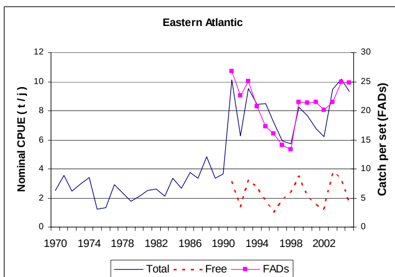
SKJ-Figura 9. Evolución de la CPUE nominal de listado de los cerqueros europeos en el Atlántico este (1970-2005). La CPUE total y la CPUE sobre banco libre se expresan en tonelada por día de pesca (eje de la izquierda) mientras que la CPUE sobre DCP se expresa en tonelada por lance positivo (eje de la derecha); la separación entre estas dos formas de pesca (banco libre vs DCP) no se ha hecho, o se ha hecho poco, en los cuadernos de pesca antes de 1990.
