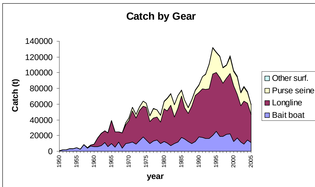
BET-Figura 1. Tendencias de las capturas de patudo (1950-2005) por principales pesquerías de túnidos.
